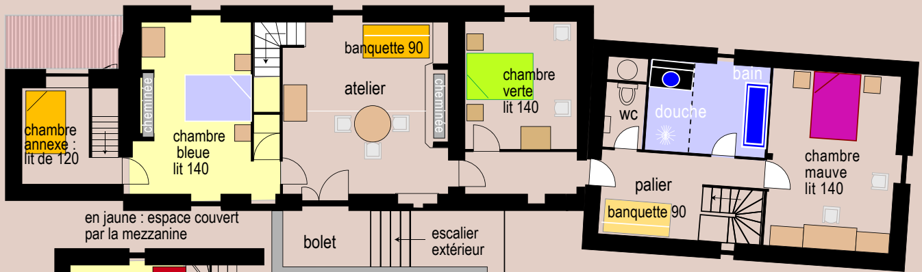
premier étage
